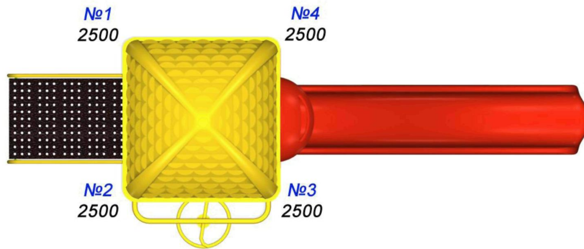
Рис. 4. Высоты площадок и опорных стоек
